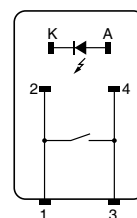
端子配置/内部连接图 (TOP VIEW)
