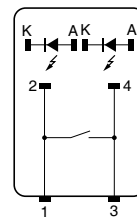
端子配置/内部连接图 (TOP VIEW)
