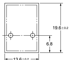
面板切割尺寸
