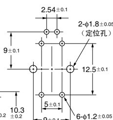
印刷基板尺寸条例 (TOP VIEW)
