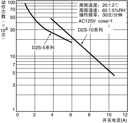
● 电气寿命曲线
