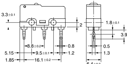
＜印刷基板用端子孔加工图（参考）＞
