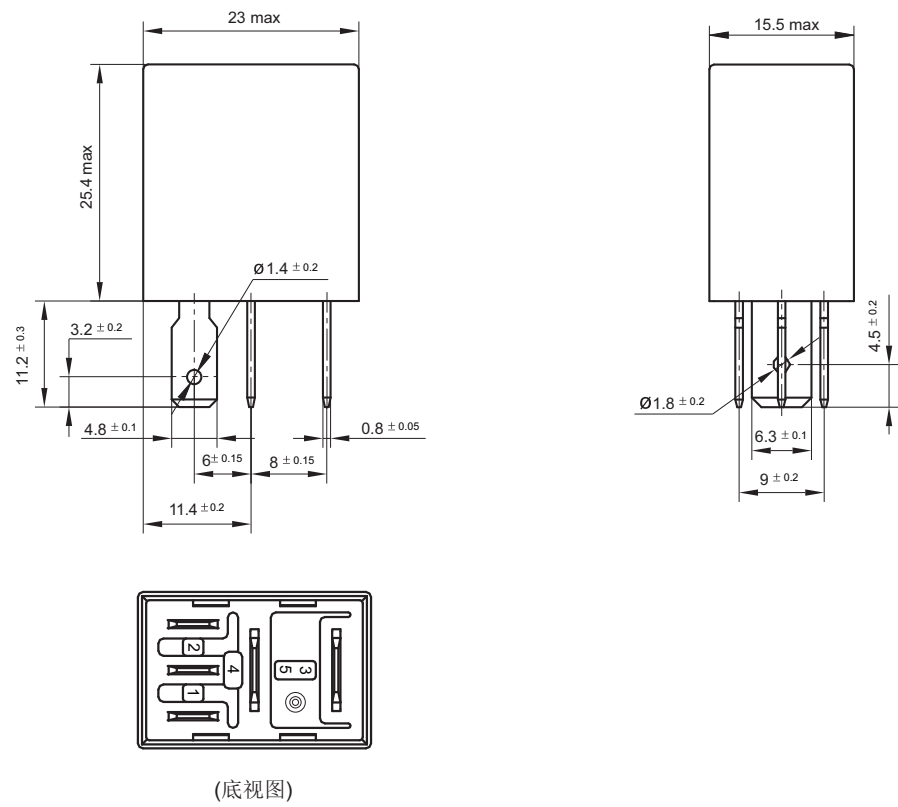
外形图
