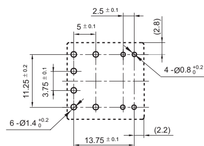
两组转换(2Z) / 双继电器
