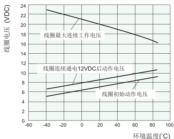
178Ω线圈连续通电电压范围
