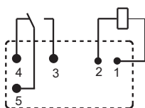
一组转换(1Z) / 单继电器
