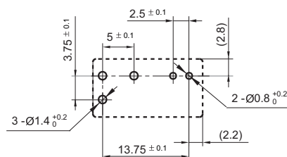
一组转换(1Z) / 单继电器
