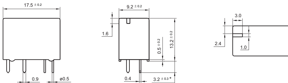
一组转换(1Z) / 单继电器
