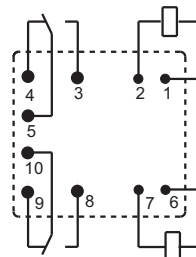
两组转换(2Z) / 双继电器
