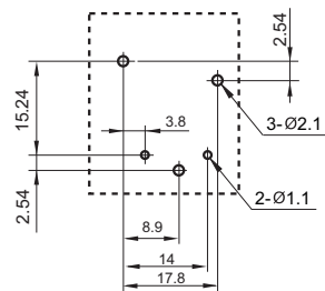
(顶视图)
