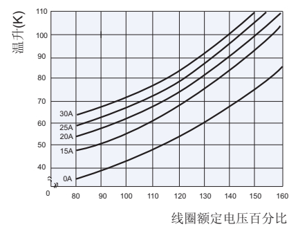
线圈温升
