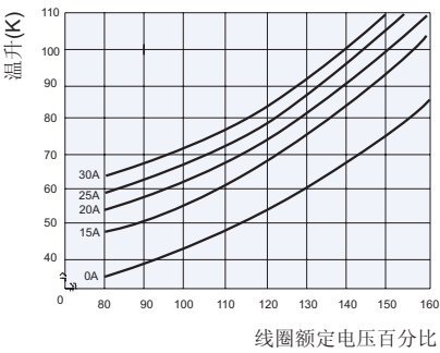
线圈温升
