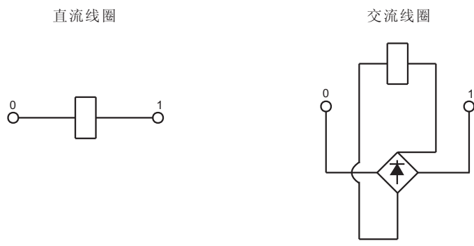
线圈接线图
