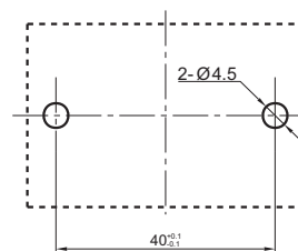
安装孔尺寸
